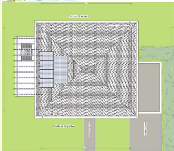
2 Pianta della Copertura - Situazione in Progetto
